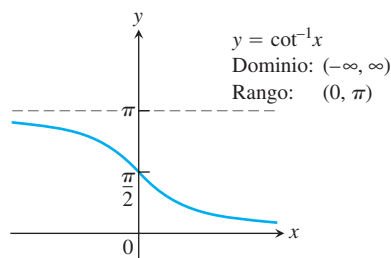
FIGURA 7.23 Gráfica de y = \cot^{-1} x .
