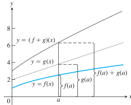
FIGURA 1.50 Suma gráfica de dos funciones.
