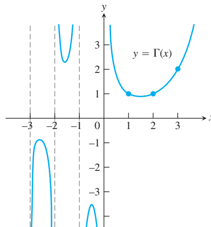
FIGURA 8.27 La función gama de Euler, \Gamma(x) es una función continua de x , cuyo valor en cada entero positivo n+1 es n! . La fórmula por medio de una integral definida para \Gamma es válida sólo para x > 0 , pero \Gamma puede extenderse a valores negativos no enteros de x con la fórmula \Gamma(x) = (\Gamma(x+1))/x , que es tema del ejercicio 49.
