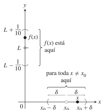
FIGURA 2.13 ¿Cómo podemos definir \delta > 0 de manera que, tomando x en el intervalo (x_0 - \delta, x_0 + \delta) f(x) se mantenga dentro del intervalo \left(L - \frac{1}{10}, L + \frac{1}{10}\right) ?
