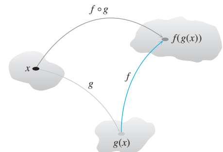
FIGURA 1.53 Diagrama de flechas para f \circ g .
