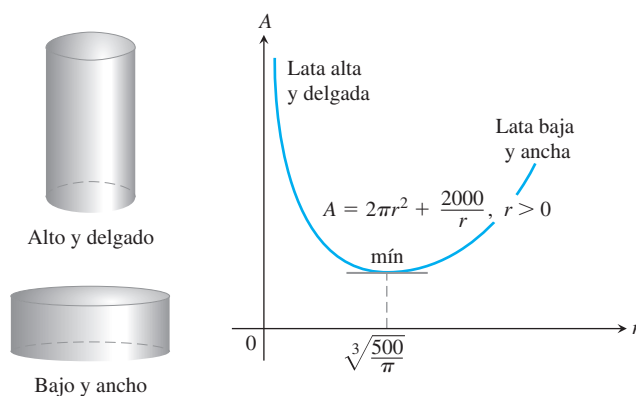
FIGURA 4.35 La gráfica de A = 2\pi r^2 + 2000/r es cóncava hacia arriba.
