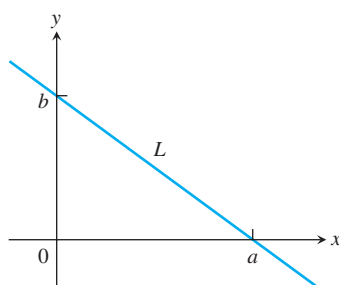
FIGURA 1.14 La recta L tiene una intersección x a y una intersección y b .
