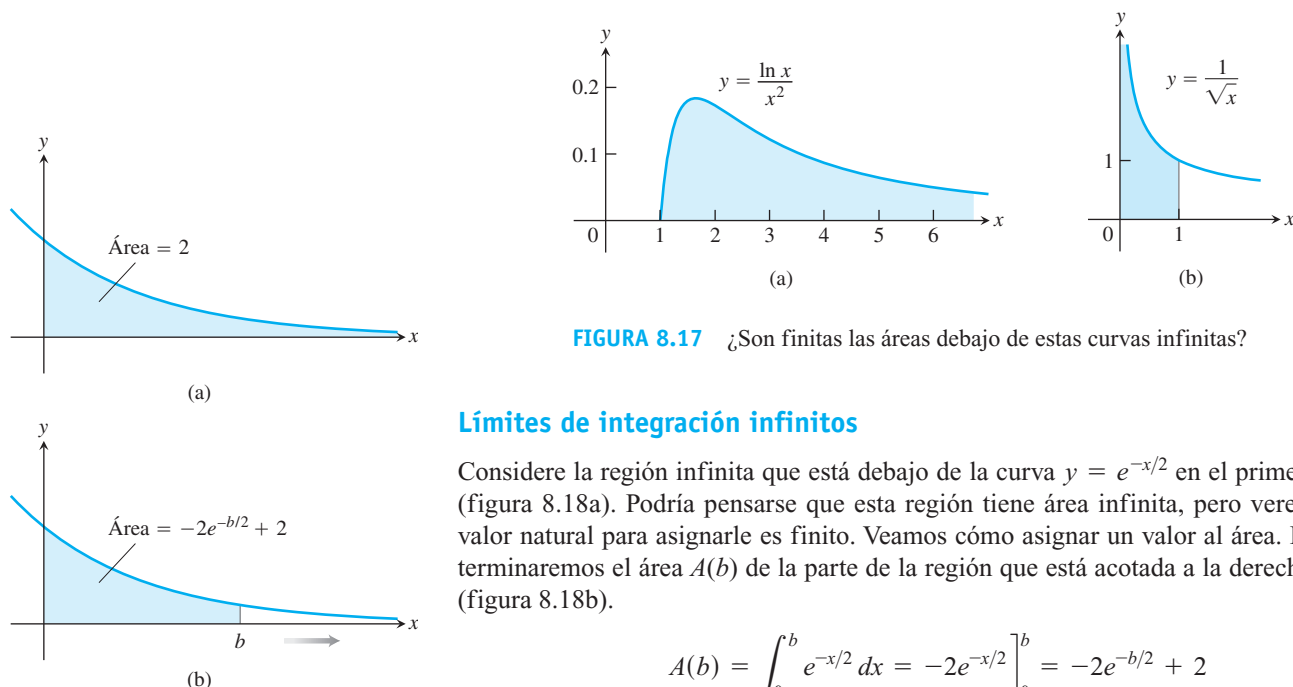
FIGURA 8.18 El área en el primer cuadrante de la curva y = e^{-x/2} es (b) una integral impropia del primer tipo.
