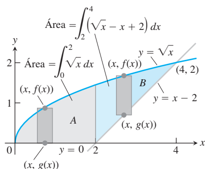
FIGURA 5.31 Cuando la fórmula para una curva frontera cambia, el área total cambia para convertirse en la suma de integrales y coincidir con aquella, una integral para cada una de las regiones sombreadas que se muestran aquí para el ejemplo 5.
