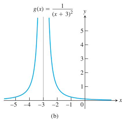
FIGURA 2.39 Las gráficas de las funciones del ejemplo 2. (a) f(x) tiende a infinito conforme x \rightarrow 0 . (b) g(x) tiende a infinito conforme x \rightarrow -3 .
