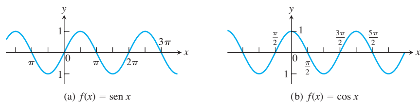
FIGURA 1.42 Gráficas de las funciones seno y coseno.
