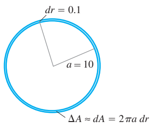
FIGURA 3.52 Cuando dr es pequeño en comparación con a , como sucede cuando dr = 0.1 y a = 10 , la diferencial dA = 2\pi a \, dr da una manera de estimar el área del círculo con radio r = a + dr (ejemplo 6).
