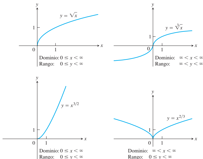
FIGURA 1.38 Gráficas de funciones de potencia f(x) = x^a para a = \frac{1}{2}, \frac{1}{3}, \frac{3}{2}, \frac{2}{3} .
