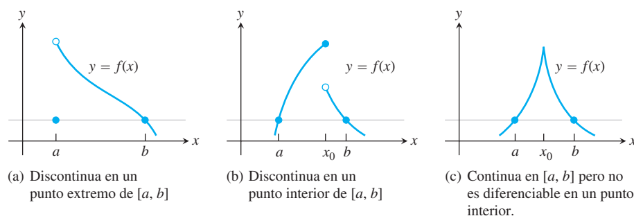
FIGURA 4.11 Puede no haber tangente horizontal si las hipótesis del teorema de Rolle no se cumplen.
