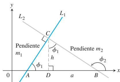
FIGURA 1.15 \triangle ADC es semejante a \triangle CDB . En consecuencia, \phi_1 también es el ángulo superior en \triangle CDB . A partir de los lados de \triangle CDB , vemos que \tan \phi_1 = a/h .
