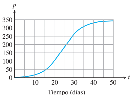
FIGURA 1.26 Gráfica de la mosca de la fruta contra el tiempo (ejemplo 3).
