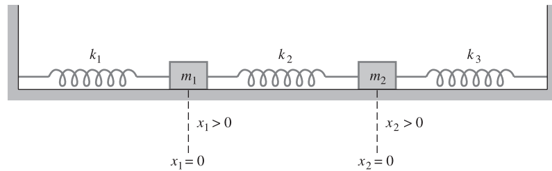
Figura 9.5 Sistema acoplado masa-resorte con extremos fijos
