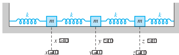
Figura 5.26 Sistema masa-resorte acoplado con tres grados de libertad
