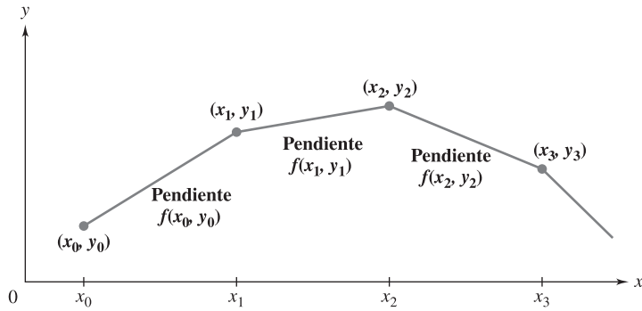
Figura 1.15 Aproximación mediante poligonales dada por el método de Euler
