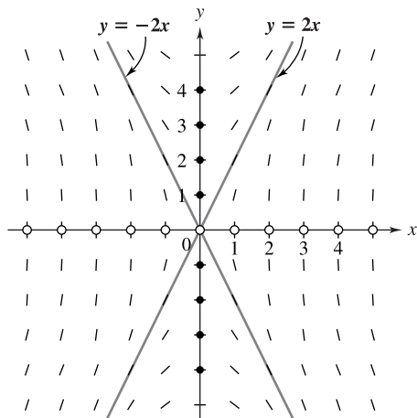
Figura 1.12 Campo de direcciones de dy/dx = 4x/y
