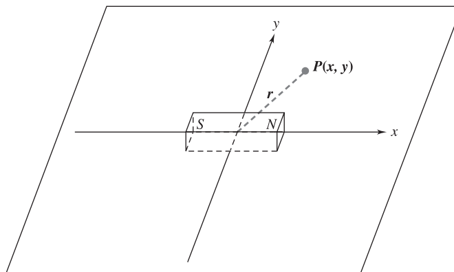
Figura 1.17 Dipolo magnético
