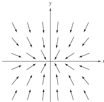
Figura 5.9 Campo de direcciones para el ejemplo 1
