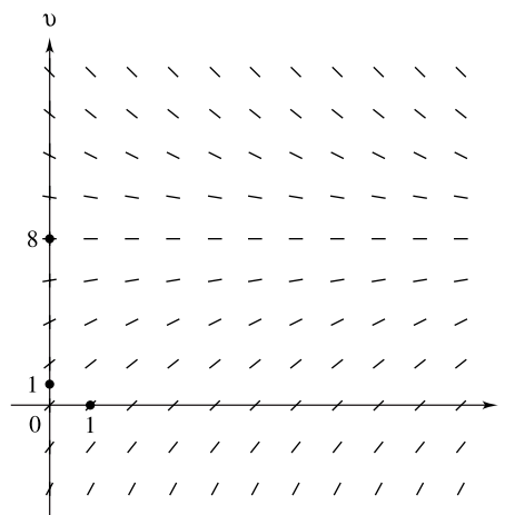
Figura 1.14 Campo de direcciones de \frac{dv}{dt} = 1 - \frac{v}{8}
