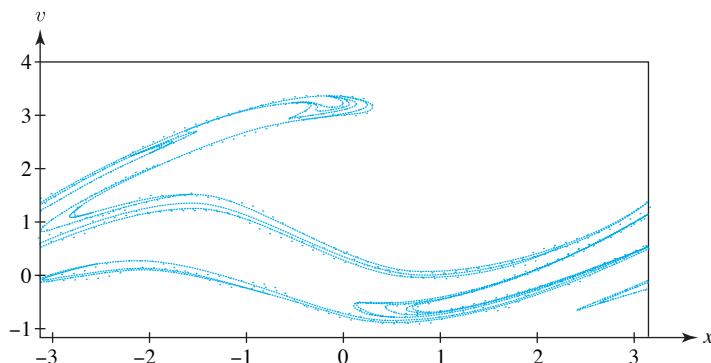
Figura 5.43 Sección de Poincaré para la ecuación del péndulo forzado (8) con b = 0.22 y F = 2.7
