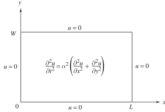
Figura 10.17 Membrana vibrante
