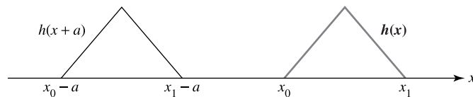
Figura 10.18 Gráficas de h(x) y h(x + a)
