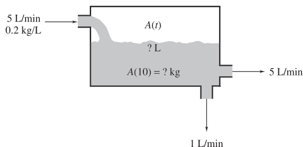
Figura 2.7 Problema de mezclas con razones de flujo distintas
