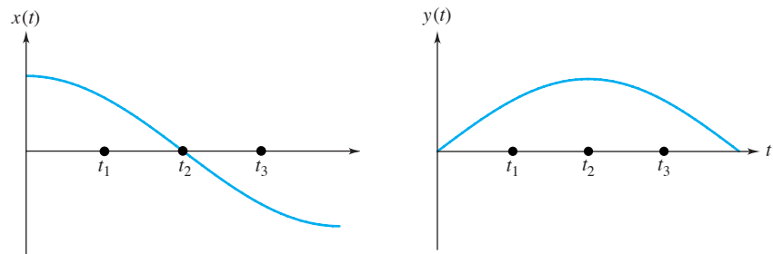
Figura 5.7 Pareja solución para el sistema (1)
